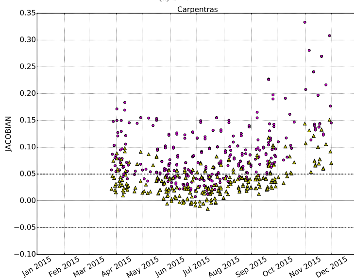
(b) PROBA-V
