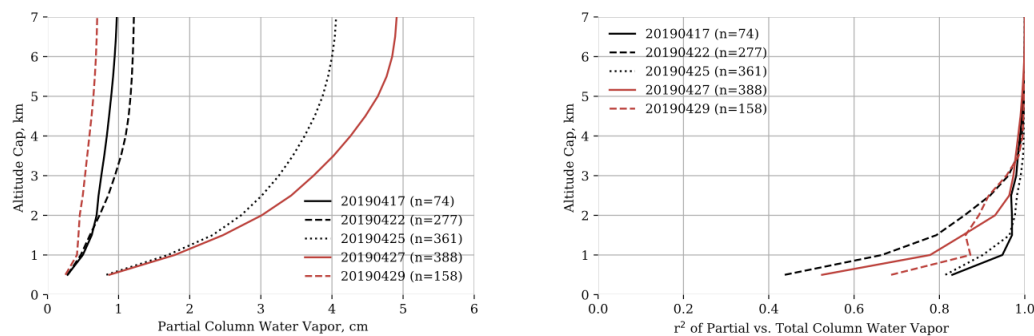
Fig. 2. Airborne Lidar Profiles
