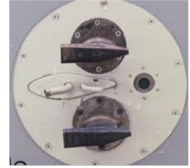
(b) MOZAIC (D-AIGI : 2001-2014)
