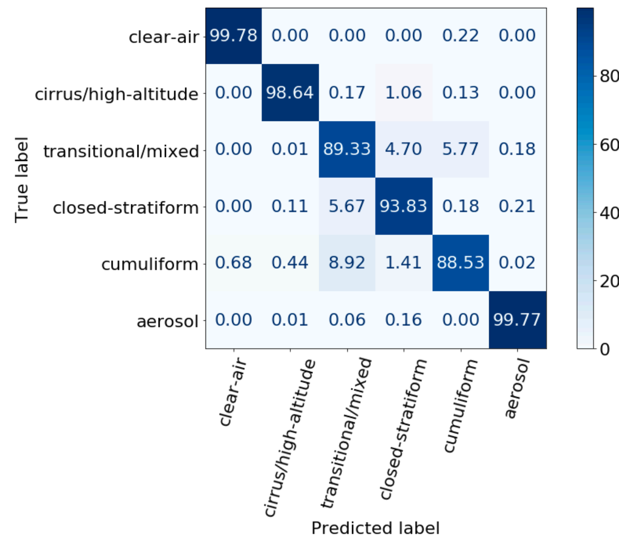
P-CNN A025
