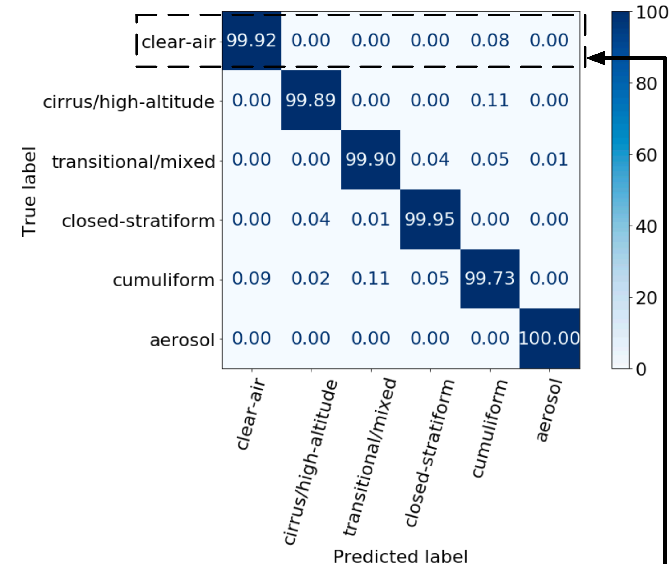
F-CNN A025
