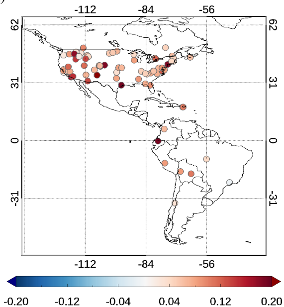
(a) ABIE DT AOD_baseline - AERONET AOD
