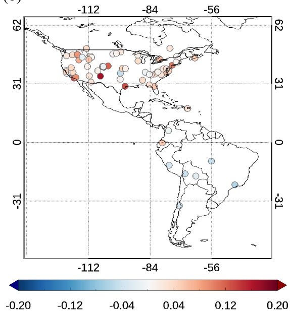
(b) ABIE DT AOD_new - AERONET AOD
