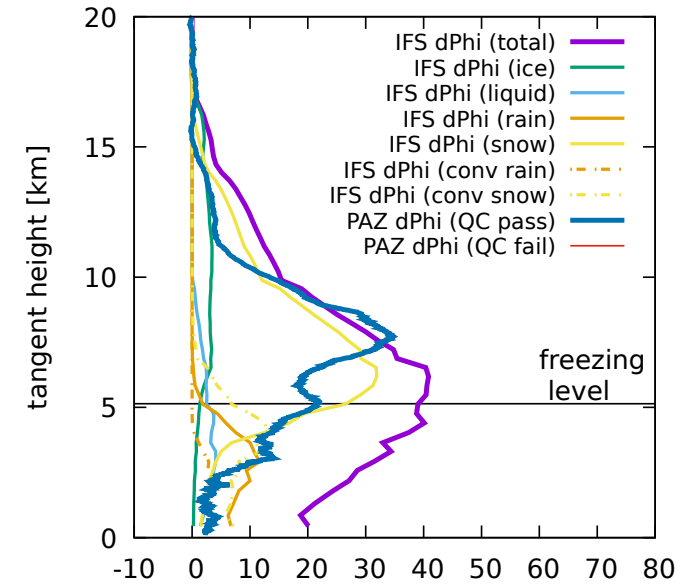
2019-10-23-BUALOI-V06-fulldrift-0.125deg
