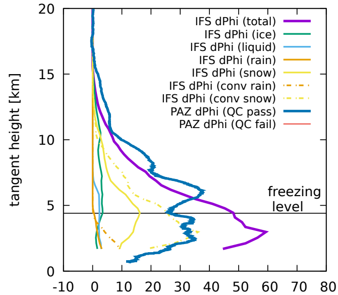
2018-05-23-MEKUNU:SAGAR-V06-fulldrift-0.125deg
