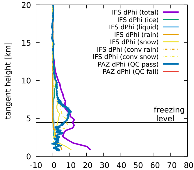
2018-10-03-LESLIE-V06-fulldrift-0.125deg
